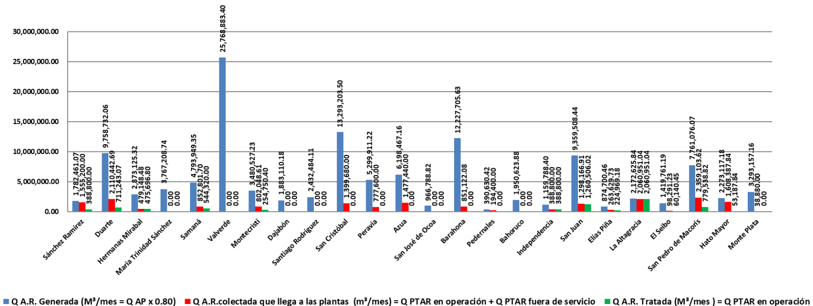
GENERACIÓN ESTIMADA DE AGUAS RESIDUALES GENERADA Vs RECOLECTADA VS TRATADA (M 3 /mes) TRIMESTRE ABRIL-JUNIO 2021
