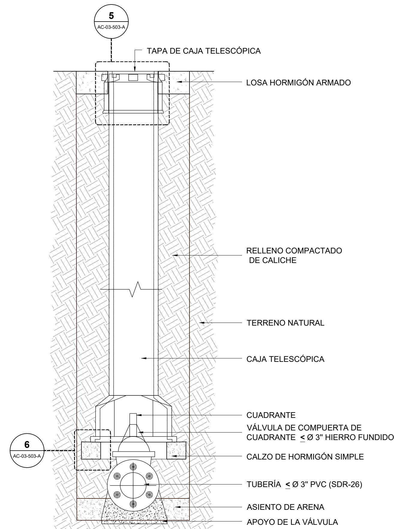
2 DETALLE CAJA TELESCÓPICA SECCIÓN A ESCALA 1:10
