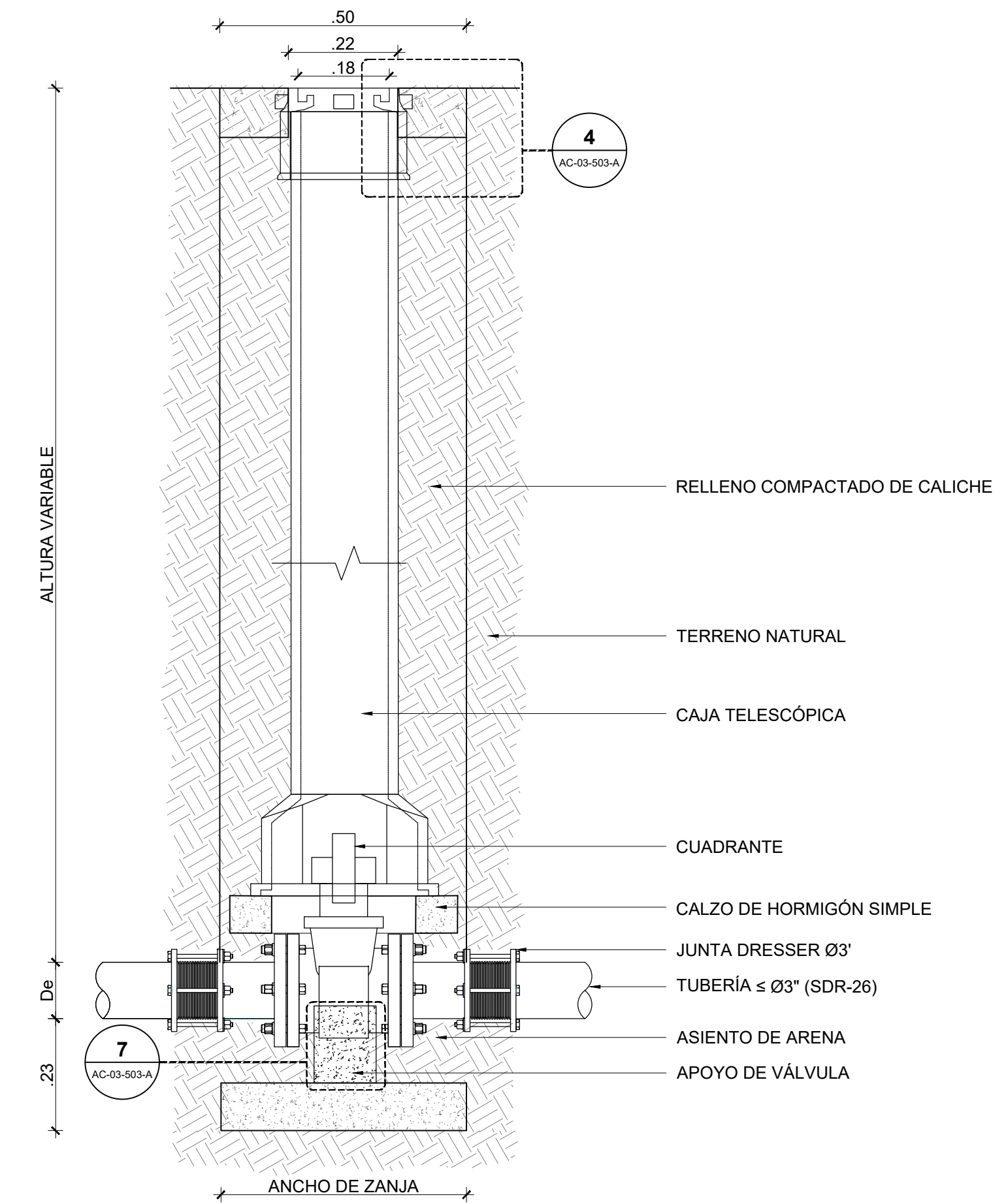
3 DETALLE CAJA TELESCÓPICA SECCIÓN B ESCALA 1:10
